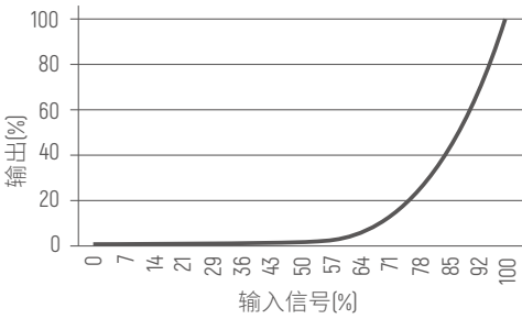
调光曲线
