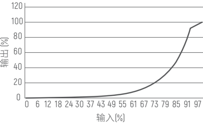
调光曲线
