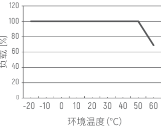
降额曲线
